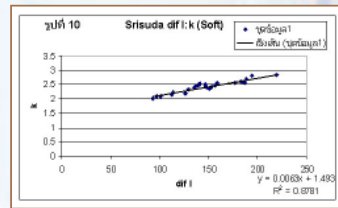
รูปที่ 1 แสดงกราฟพล็อตระหว่างค่า k ในสมการ W = kI^2R กับค่า ผลต่างของอัตราการไหลของลมที่คำนวณได้กับที่วัดได้จากเครื่อง Spirometer ( dif I ) ขณะอาสาสมัครเปล่งเสียงดัง 3 เสียงได้แก่ /i/ /a/ /u/ ใน 3 ระดับเสียงคือ สูง กลาง ต่ำอย่างละ 3 ครั้ง ครั้งละ 8-10 วินาที จะเห็นว่าความสัมพันธ์ของพารามิเตอร์ทั้ง 2 เป็นเส้นตรง และผลต่างของอัตราการไหลของลมที่คำนวณ ได้กับที่วัดได้จากเครื่อง Spirometer มีทั้งค่าบวกและลบ
