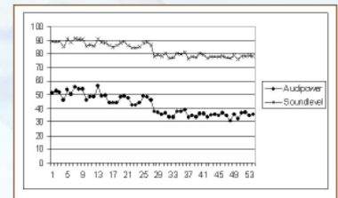
รูปที่ 2 แสดงกราฟพล็อตค่าความเข้มเสียงที่คำนวณได้จาก สัญญาณเสียงที่บันทึกด้วย Condenser Microphone (Audiotape) เทียบกับค่าที่วัดได้จากเครื่องวัดระดับเสียง meter ขณะอาสาสมัครเปล่งเสียงดังและเบา 3 เสียงได้แก่ /i/ /a/ /u/ ใน 3 ระดับเสียงคือ สูง กลาง ต่ำ อย่างละ 3 ครั้ง ครั้งละ 8-10 วินาที
