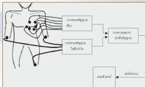
รูปที่ 1 รูปแบบเครื่องมือที่ต้องการพัฒนาขึ้น
